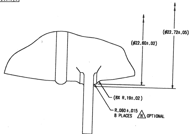
VIEW A SCALE: 2/1
