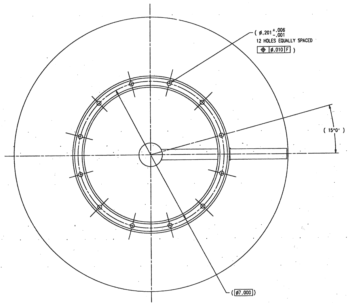
VIEW A-A
