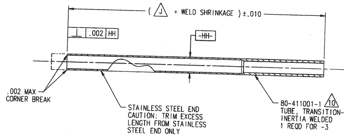
DETAIL -3 SCALE: 2/1
